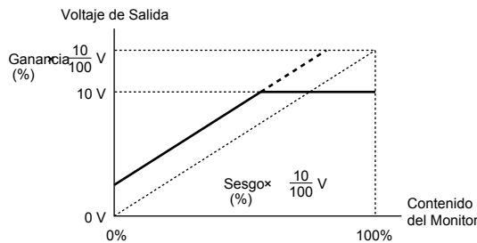
4.26 Ajuste de la Salida del Monitor
