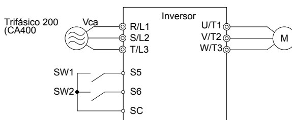
4.32 Terminales de Control para Velocidades de 4 Pasos Múltiples
