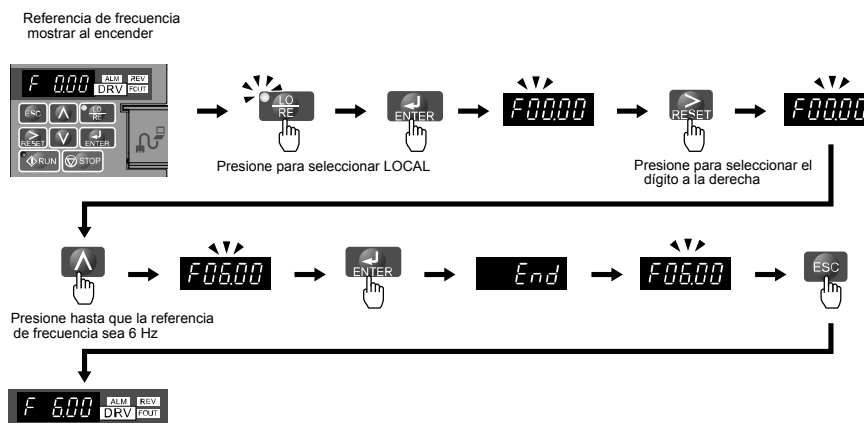
4.4 Configuración de la Referencia de Frecuencia en Modo de Inversor
