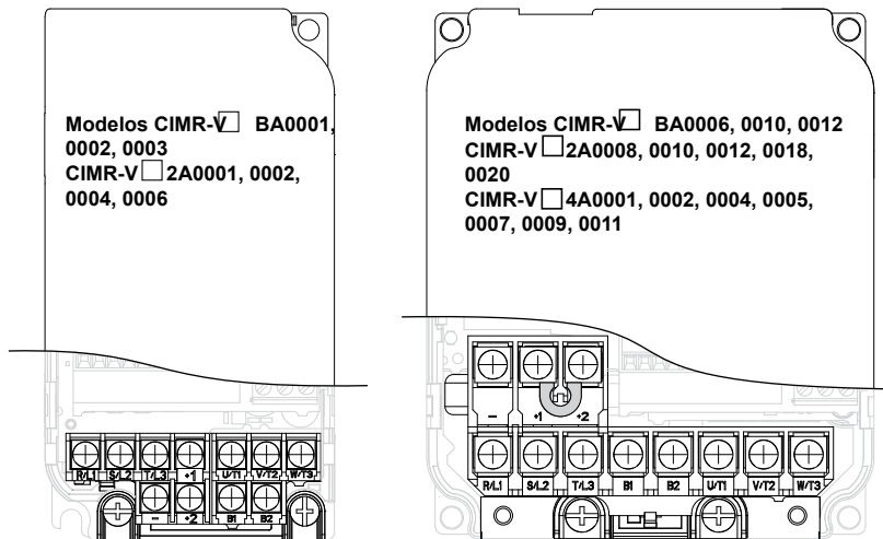
3.5 Configuraciones del Bloque de Terminales del Circuito Principal
