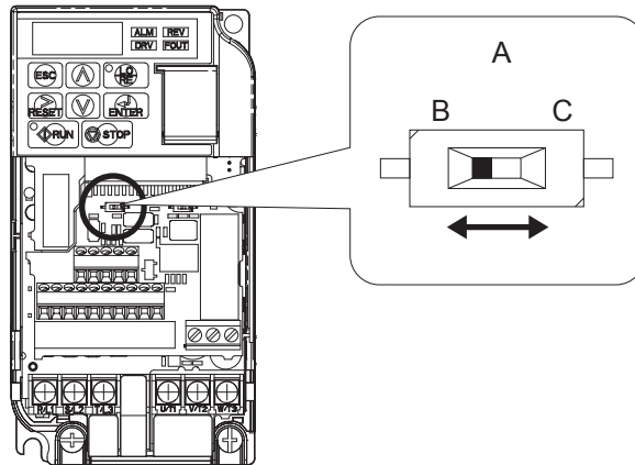
C.3 Interruptor de Terminales MEMOBUS/Modbus y Resistor Terminal
