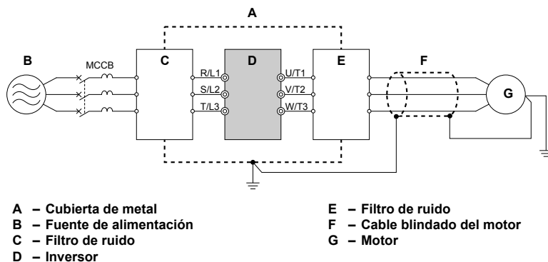
7.10 Reducción del ruido de radiofrecuencia
