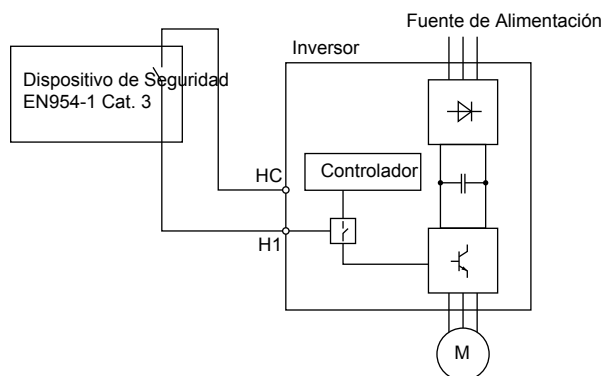
D.9 Ejemplo de Cableado de Desactivación Segura
