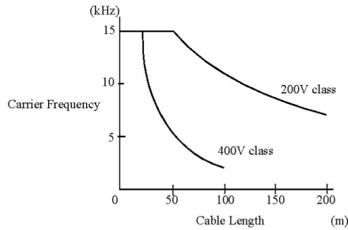
7.15 Criterios para establecer la Frecuencia de la Portadora
