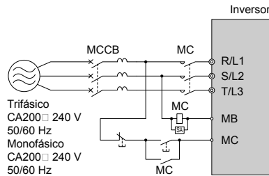
7.2 Conexión de un MCCB (para clase de 200 V trifásico)
