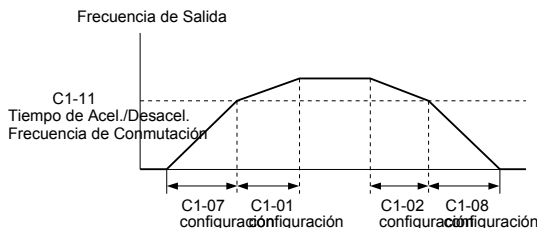
Cuando la frecuencia de salida alcanza el valor configurado en C1-11, el inversor usa el Tiempo de Acel./Desacel. 1 (C1-01). Cuando la frecuencia de salida alcanza el valor configurado en C1-11, el inversor usa el Tiempo de Acel./Desacel. 2 (C1-07, -08)
