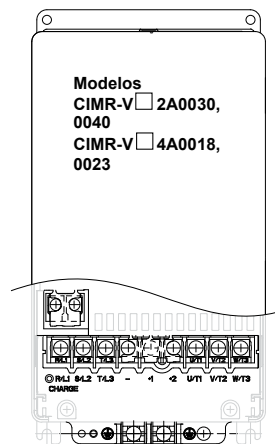
3.7 Configuraciones del Bloque de Terminales del Circuito Principal
