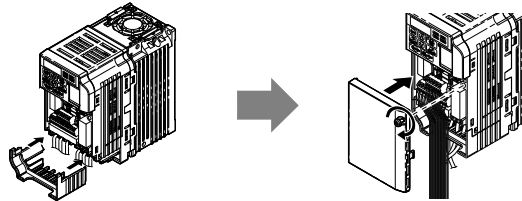
3.12 Coloque de nuevo las Tapas Protectoras en un inversor IP20/Chasis Abierto
