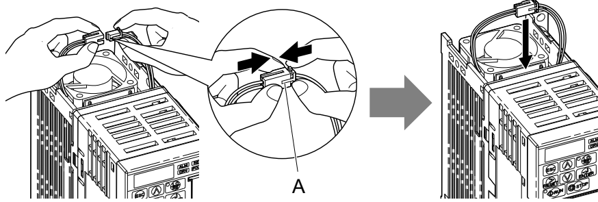
A - Junte los conectores empujándolos para que no quede espacio entre ellos.
