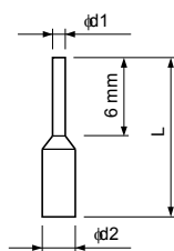
3.22 Dimensiones del Casquillo
