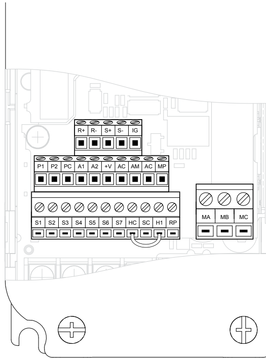
C.4 Configuración del Bloque de Terminales del Circuito de Control (CIMR-VA□□□□□□□□; CIMR-VU□□□□□□□□)
