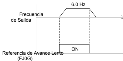
4.31 Patrón de Operación de Avance Lento
