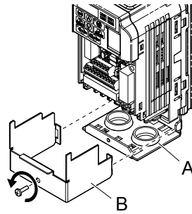
3.14 Cómo quitar la Tapa de la Terminal en un Inversor IP20/NEMA Tipo 1
