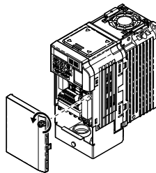
3.13 Cómo quitar la Tapa Frontal en un Inversor IP20/NEMA Tipo 1
