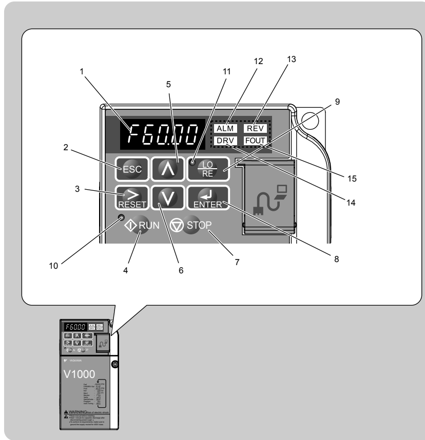
4.1 Teclas y Pantallas en el Operador LED
