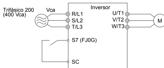
4.30 Comando de Avance Lento desde Terminales Externas
