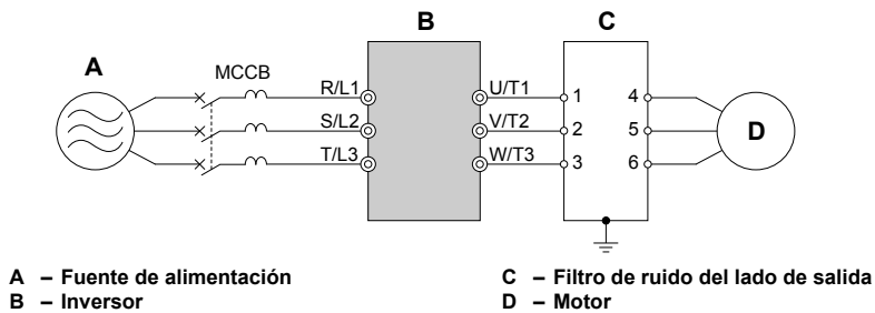
7.8 Filtro de Ruido del Lado de Salida
