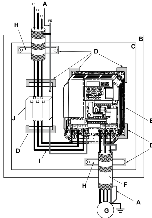
7.12 Área de Conexión a Tierra
