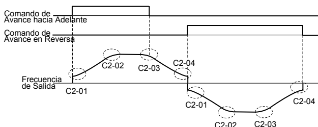
4.22 Características de Curva S
