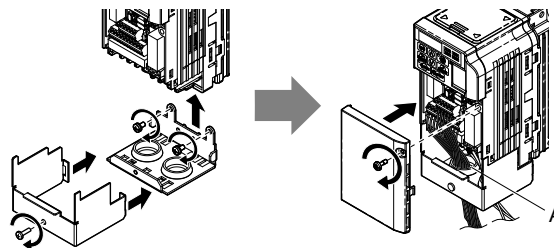
3.16 Cómo colocar de nuevo las Tapas Protectoras y el Soporte del Conducto en un Inversor IP20/NEMA Tipo 1
