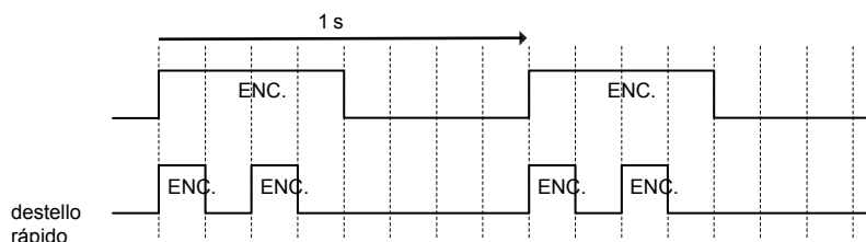
4.1 Estado y significado del LED RUN
