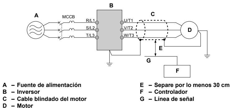
7.9 Cómo evitar el Ruido Inducido
