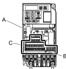
6.4 Tablero de Terminales
