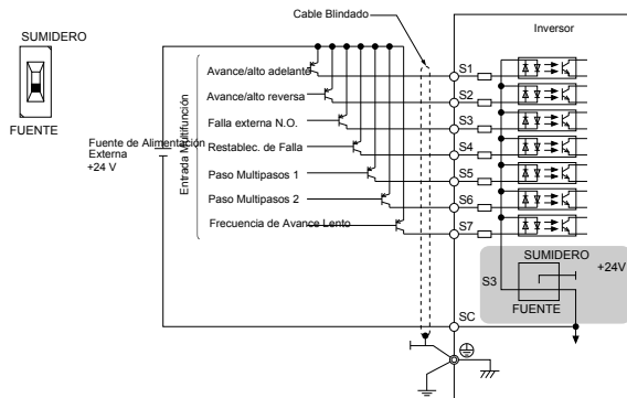
3.28 Modo de Fuente: Secuencia desde Transistor PNP (Común de +24 V)
