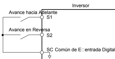
4.15 Diagrama de Cableado de Ejemplo para Secuencia de 2 cables
