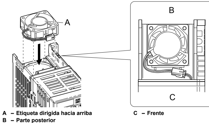
6.2 Orientación del Ventilador de Enfriamiento
