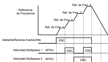
4.33 Gráfica de Tiempo de Velocidad de 4 Pasos
