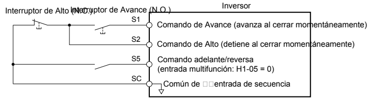
3.2 Secuencia de 3 Hilos
