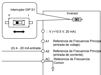
4.13 Entrada de Corriente para la Referencia de Frecuencia Principal
