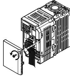
3.10 Cómo quitar la tapa frontal de un inversor IP20/Chasis Abierto
