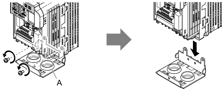
3.15 Cómo quitar la Tapa de la Terminal en un Inversor IP20/Chasis Abierto
