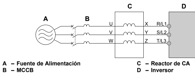
7.4 Conexión de un Reactor de CA
