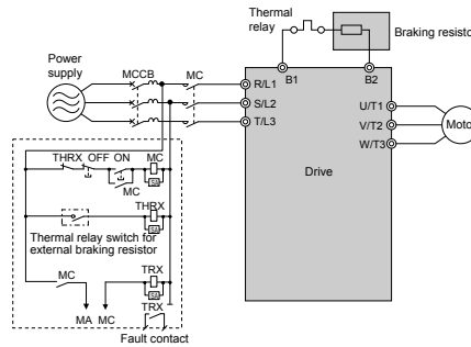
3.31 Conexión de un Resistor de Frenado
