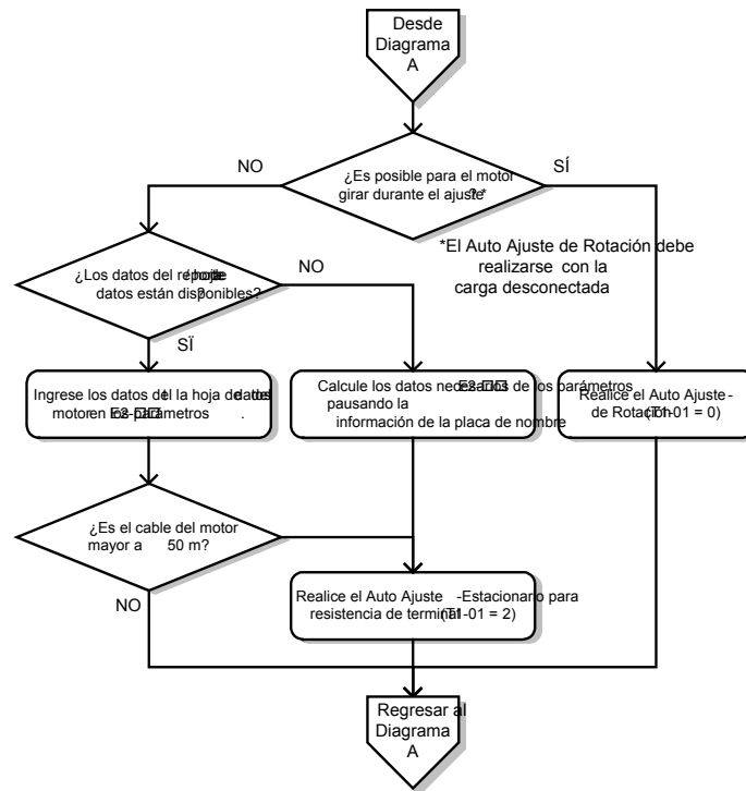
4.8 Diagrama de Flujo A2: Operación de Alto Desempeño Usando Control de Motor de Vector de Ciclo Abierto
