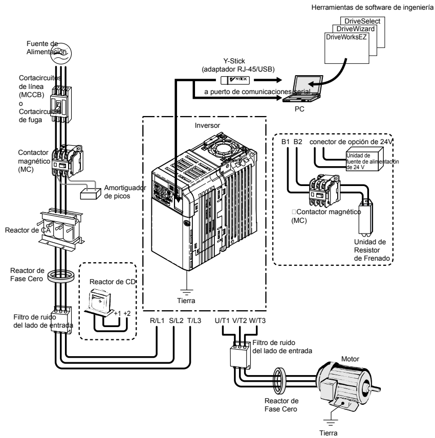
7.1 Conexión de dispositivos periféricos
