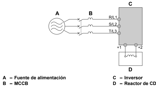
7.5 Conexión de un Reactor de CD
