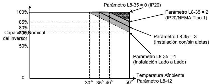
A.2 Reducción de Potencia de Método de Instalación y Temperatura Ambiente
