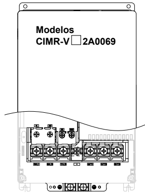
3.9 Configuraciones del Bloque de Terminales del Circuito Principal
