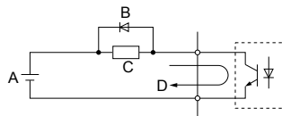
A – Alimentación externa, 48 V máx. C – Bobina B – Diodo supresor D – 50 mA o menor
