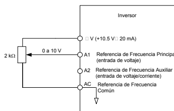
4.12 Entrada de Voltaje para la Referencia de Frecuencia Principal
