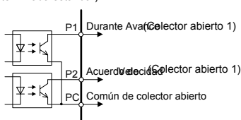
4.25 Diagrama de Conexión de Salida Digital
