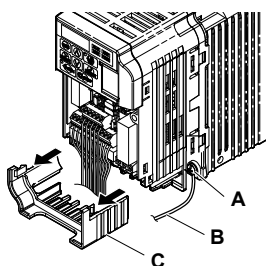
7.18 Conecte el cable
