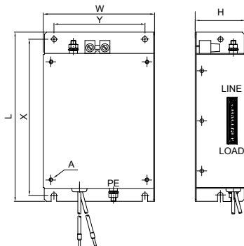
D.6 Dimensiones de un Filtro EMC
