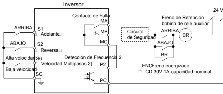
4.10 Diseño del Circuito del Freno de Retención
