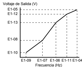
4.24 Patrón de V/f
