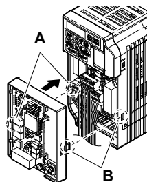
7.19 Conecte la tarjeta de opción
