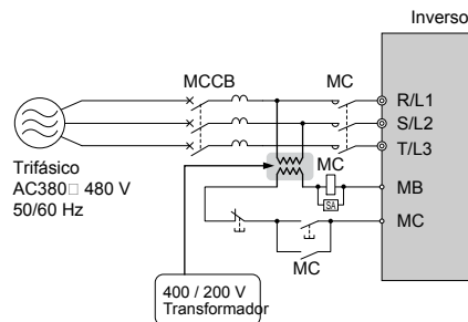
7.3 Conexión de un MCCB (para clase de 200 V trifásico)
