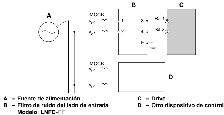
7.6 Filtro de ruido del lado de entrada (Monofásico 200 V)
