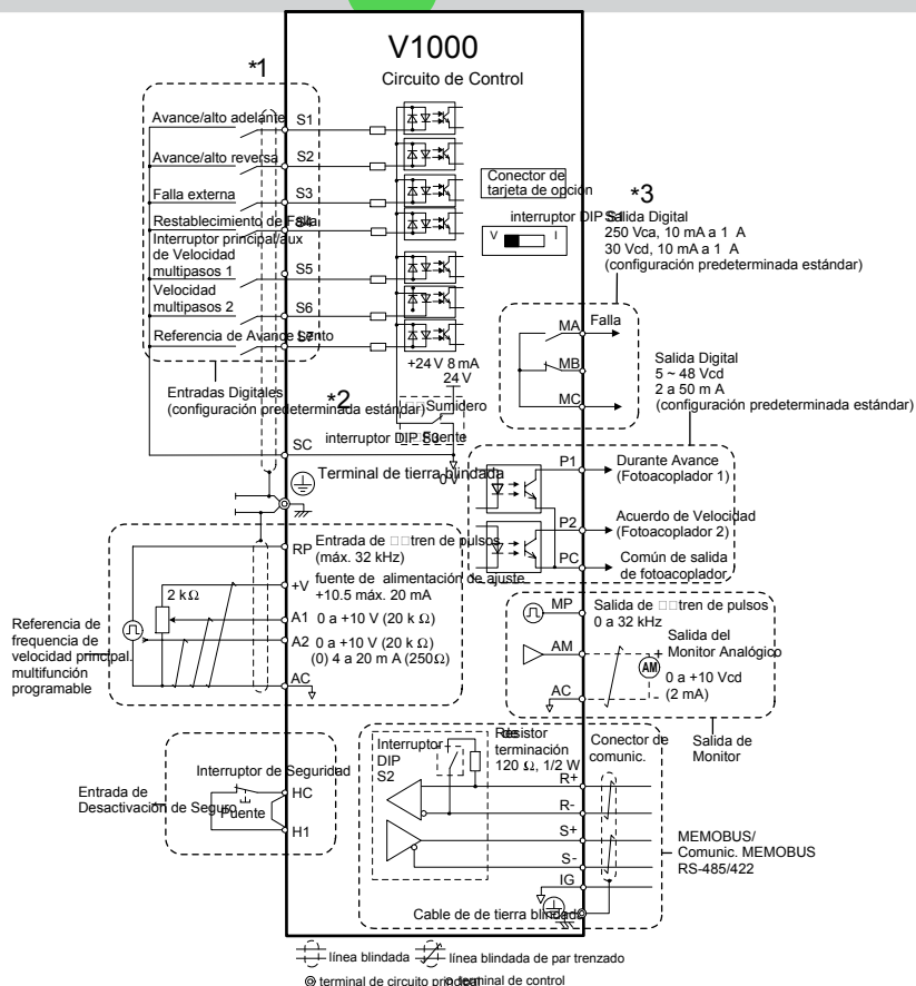
3.19 Diagrama de Cableado del Circuito de Control
