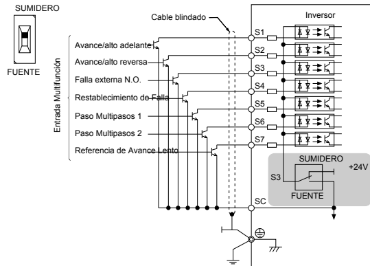
3.27 Modo de Sumidero: Secuencia desde Transistor NPN (Común de 0 V)
