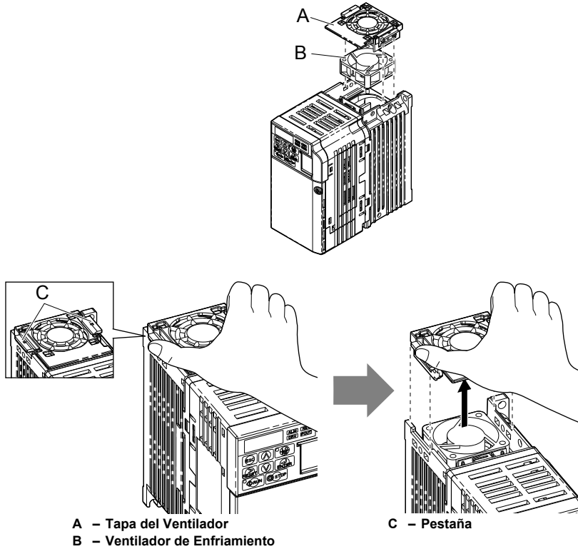
6.1 Quite la Tapa del Ventilador de Enfriamiento
