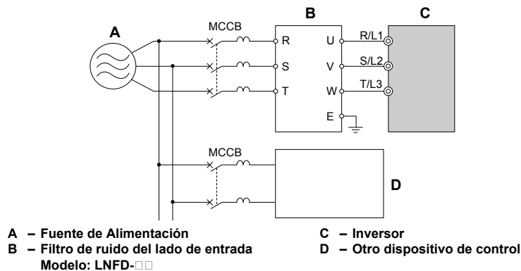
7.7 Filtro de ruido del lado de entrada (Trifásico 200/400 V)
