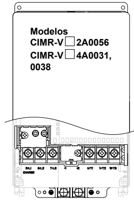
3.8 Configuraciones del Bloque de Terminales del Circuito Principal
