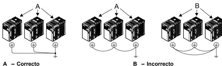
3.17 Cableado de Varios Inversores
