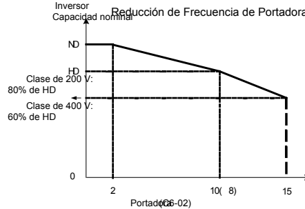
A.1 Reducción de la Frecuencia de la Portadora
