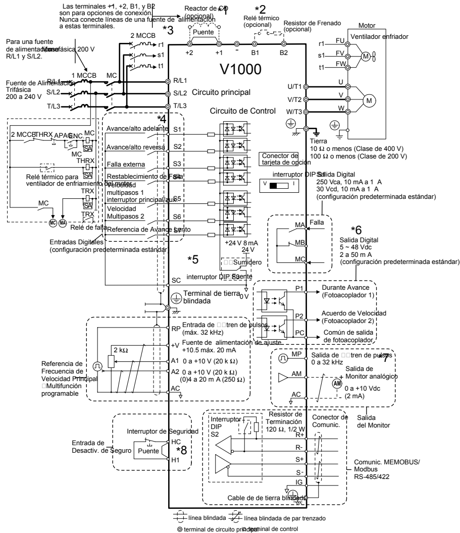
3.1 Diagrama de Conexión Estándar del Inversor
