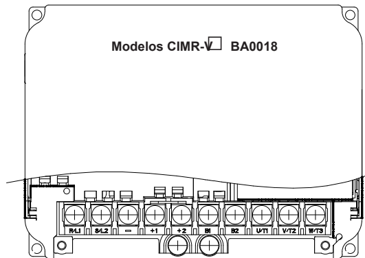
3.6 Configuraciones del Bloque de Terminales del Circuito Principal
