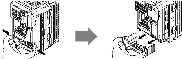
3.11 Quite la Tapa de la Terminal en un Inversor IP20/Chasis Abierto
