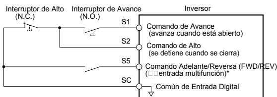
4.16 Diagrama de Cableado de Ejemplo para una Secuencia de 3 cables Usando una Terminal S5
