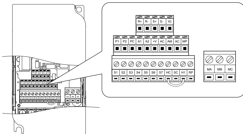
3.21 Bloque de Terminales del Circuito de Control Removible (CIMR-VC□□□□□□□□□□; CIMR-VAZ□□□□□□□□□□)
