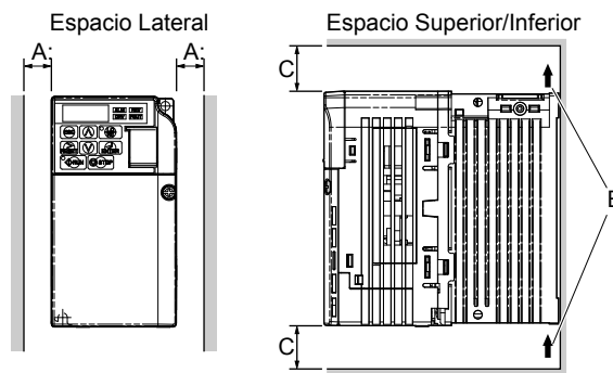
A – 30 mm mínimo
